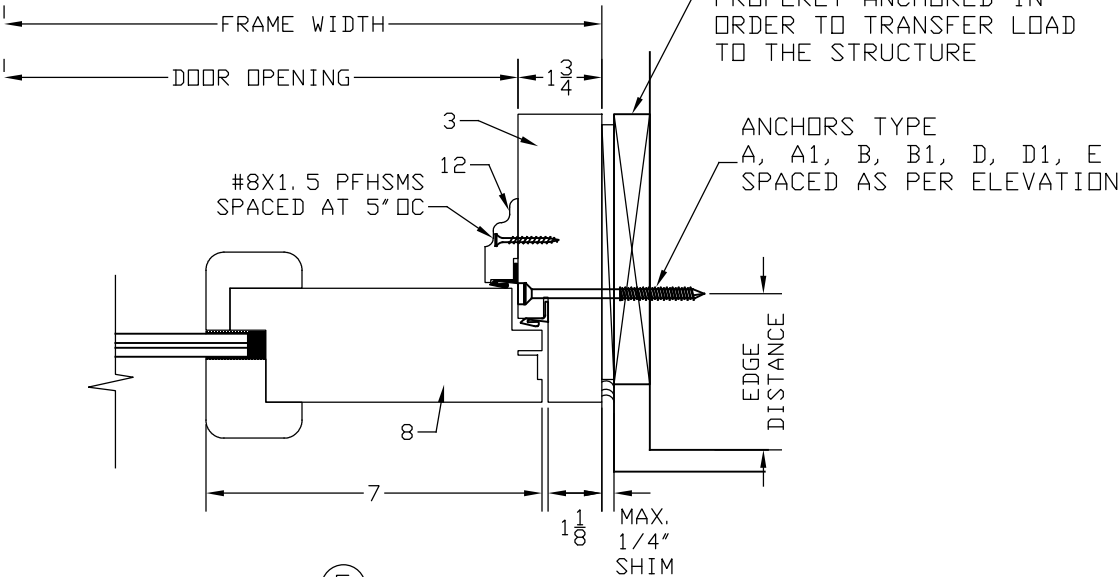
(E) JAMB LOCK
