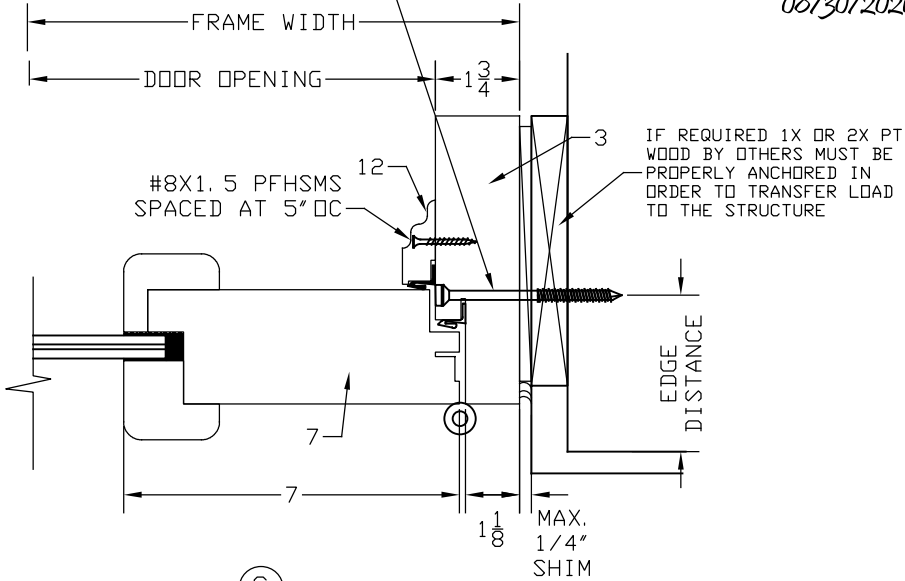
(C) JAMB HINGE
